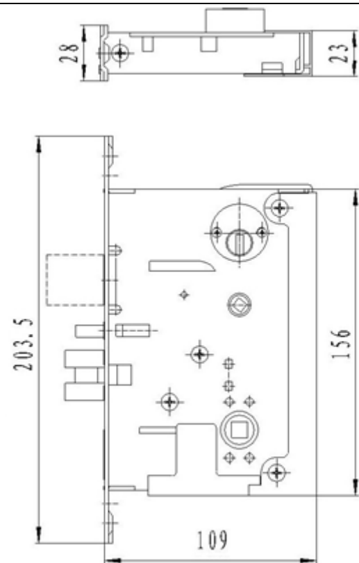
Размеры врезного механизма замка
